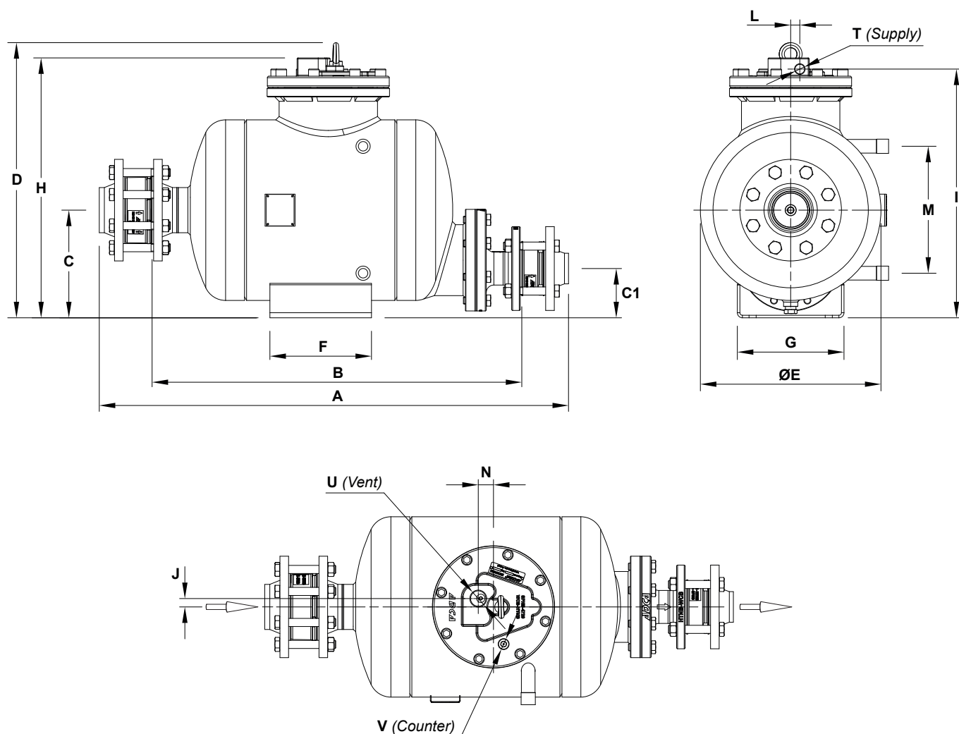
DIMENSIONS – PN 16 (mm)
